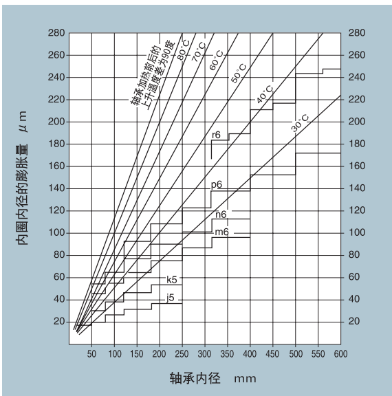
内圈热嵌装所必须的加热温度
